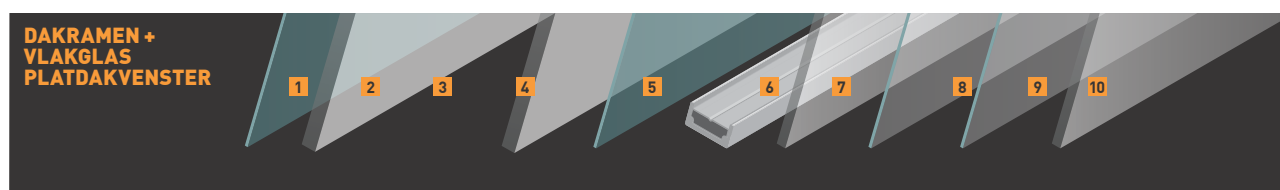
1, 4: 3 mm floatglas 2, 3: Twee lagen van scheurbestendige folie 5: Met argon gevulde holte 6: Warmtereflecterende lage-emissiecoating 7: 4 mm floatglas 8: 32 mm geventileerde spleet tussen basis en koepel van platdakvenster 9: 4 mm gehard glas 10: Eenvoudig te reinigen coating
