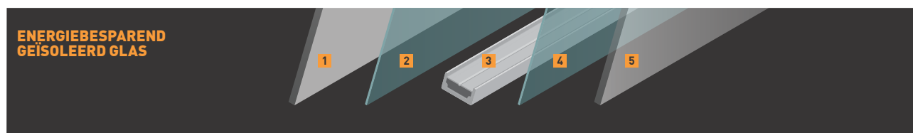
1: 4 mm gehard veiligheidsglas 2, 4: Lage-emissiecoating [reflecteert warmte] 3: Vulling met Argon gas 5: 4 mm floatglas
